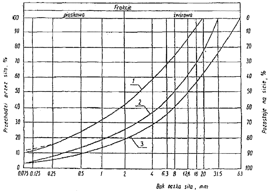
Rysunek 1. Pole dobrego uziarnienia kruszyw przeznaczonych na podbudowy wykonywane metodą stabilizacji mechanicznej 1-2 kruszywo na podbudowę zasadniczą 1-3 kruszywo na podbudowę pomocniczą
